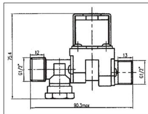
Рис.2. Установочные размеры.
