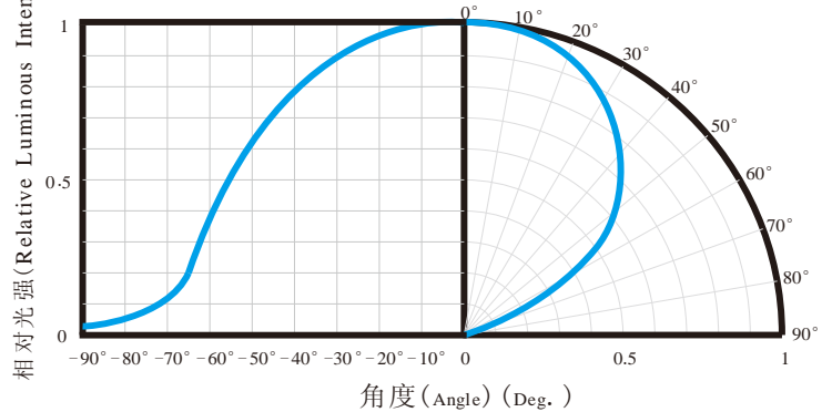
光强分布特性曲线 Typical Spatial Distribution
